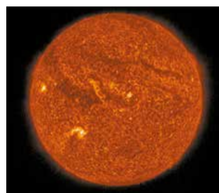
У Солнца зернистая поверхность. Фото 28 июля 2016 г.
