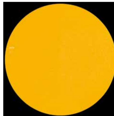
28 июля 2016 года. Пятен нет. Активность близка к нулю. Это фото в белом свете
