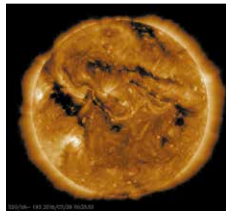
Солнечная корона 28 июля в ином спектре
