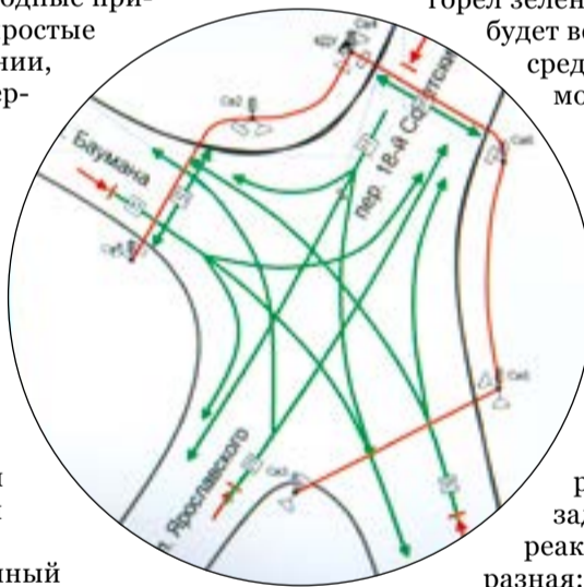
Схема организации дорожного движения на перекрестке: зеленым обозначено направление движения, красным — кабельные трассы
