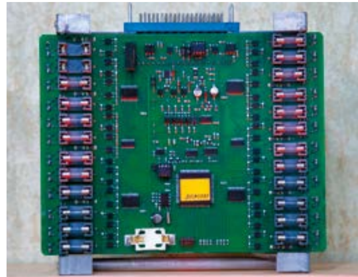
Дорожный контроллер — сердце светофора, именно он управляет всеми тремя сигналами: красным, желтым, зеленым
