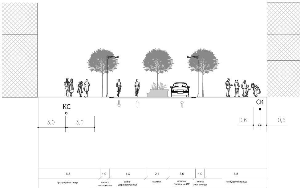
Строительство (перенос) ул. Подгорная (сечение разреза 10-10) 11 метров
