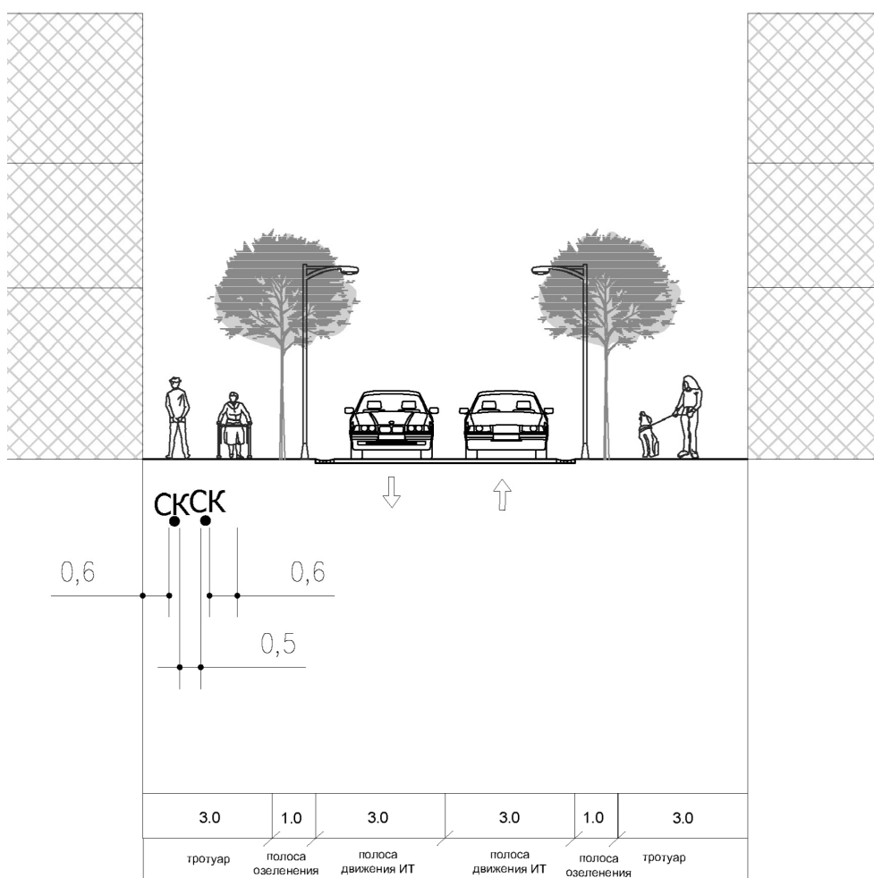
Раздел 3. Поперечные профили улиц и магистралей Реконструкция ул. Лапина (сечение разреза 11-11) 14 метров
