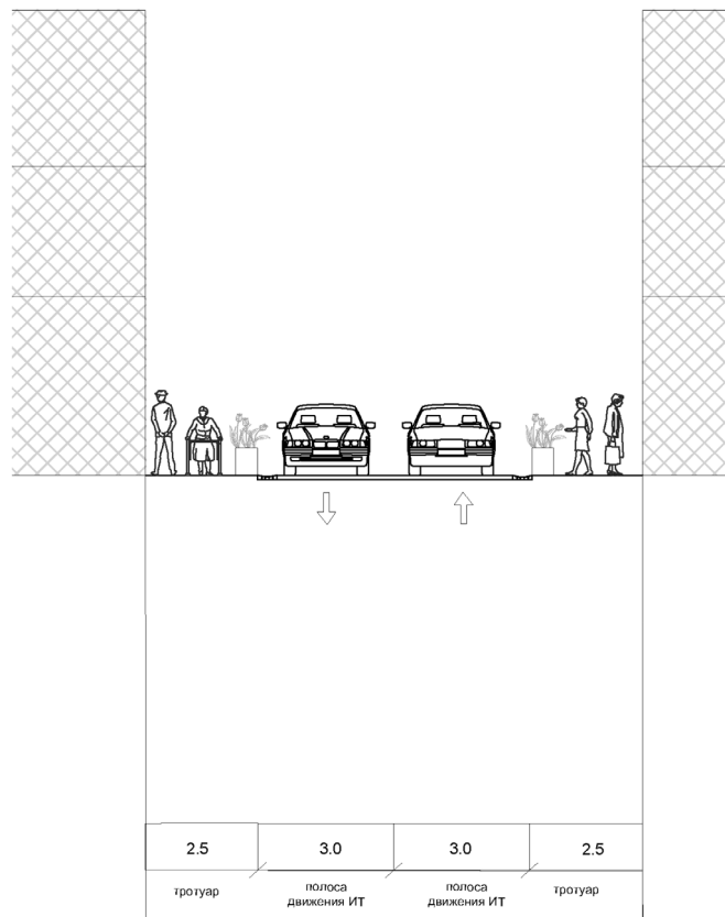
Строительство (перенос) ул. Подгорная (сечение разреза 10-10) 11 метров
