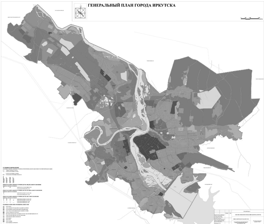
КАРТА ПЛАНИРУЕМОГО РАЗМЕЩЕНИЯ ОБЪЕКТОВ МЕСТНОГО ЗНАЧЕНИЯ ГОРОДСКОГО ОКРУГА. ЭЛЕКТРОСНАБЖЕНИЕ.
