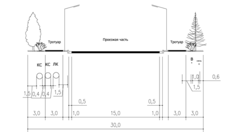
МАГИСТРАЛЬНАЯ УЛИЦА ОБЩЕГОРОДСКОГО ЗНАЧЕНИЯ РЕГУЛИРУЕМОГО ДВИЖЕНИЯ. СВЯЗКА УЛИЦЫ ОЛЕГА КОШЕВОВО И УЛИЦЫ ВОРОСКОГО (СЕЧЕНИЕ РАЗРЕЗА 4-4)
