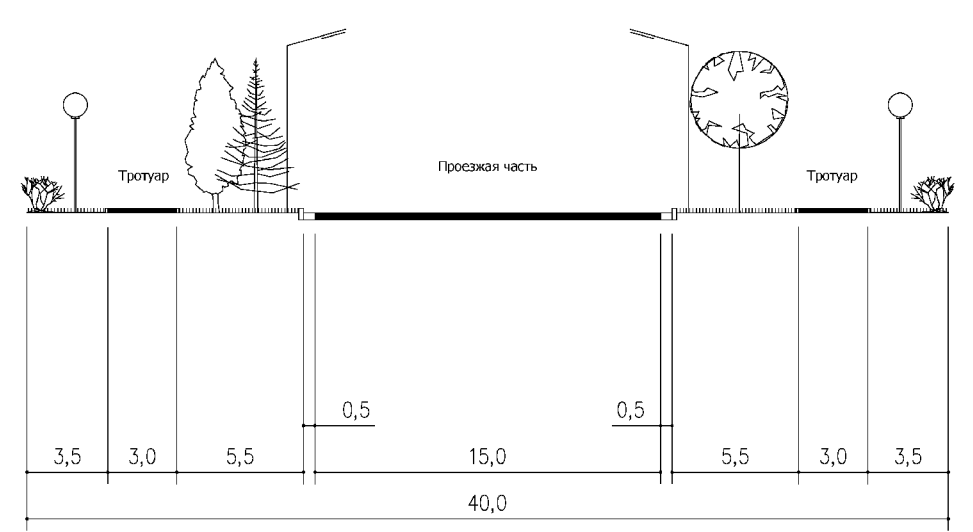
МАГИСТРАЛЬНАЯ УЛИЦА ОБЩЕГОРОДСКОГО ЗНАЧЕНИЯ РЕГУЛИРУЕМОГО ДВИЖЕНИЯ. УЛИЦА ВОРОВСКОГО (СЕЧЕНИЕ РАЗРЕЗА 2-2)
