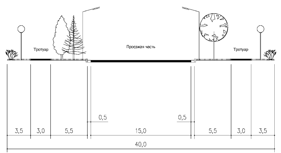
1.3. ПОПЕРЕЧНЫЕ ПРОФИЛИ УЛИЦ И ДОРОГ В КРАСНЫХ ЛИНИЯХ МАГИСТРАЛЬНАЯ ДОРОГА РЕГУЛИРУЕМОГО ДВИЖЕНИЯ. УЛИЦА ПОЛЯРНАЯ (СЕЧЕНИЕ РАЗРЕЗА 1-1)
