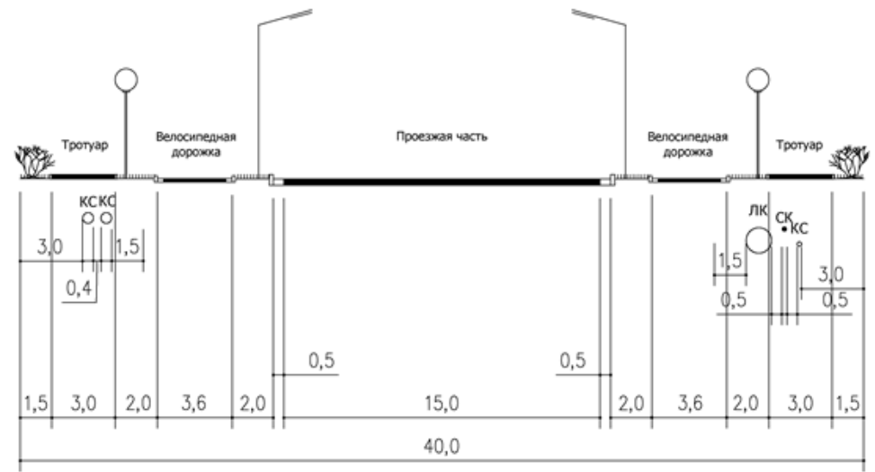
МАГИСТРАЛЬНАЯ УЛИЦА РАЙОННОГО ЗНАЧЕНИЯ. УЛИЦА ДАЛЬНЕВОСТОЧНАЯ (УЧАСТОК ПАРАЛЛЕЛЬНЫЙ УЛ. БАЙКАЛЬСКОЙ), СЕЧЕНИЕ РАЗРЕЗА 2-2
