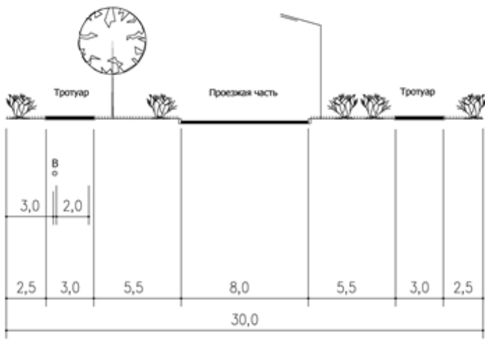
УЛИЦА МЕСТНОГО ЗНАЧЕНИЯ. СЕЧЕНИЕ РАЗРЕЗА 4-4
