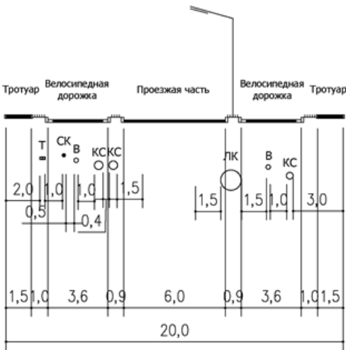
УЛИЦА МЕСТНОГО ЗНАЧЕНИЯ. УЛИЦА ВЕРХНЯЯ НАБЕРЕЖНАЯ, СЕЧЕНИЕ РАЗРЕЗА 3-3
