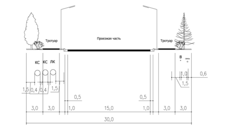
УЛИЦА МЕСТНОГО ЗНАЧЕНИЯ (СЕЧЕНИЕ РАЗРЕЗА 5-5)
