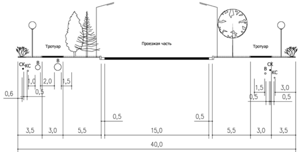
МАГИСТРАЛЬНАЯ УЛИЦА РАЙОННОГО ЗНАЧЕНИЯ. УЛИЦА ДАЛЬНЕВОСТОЧНАЯ (УЧАСТОК ПАРАЛЛЕЛЬНЫЙ УЛ. БАЙКАЛЬСКОЙ), СЕЧЕНИЕ РАЗРЕЗА 2-2
