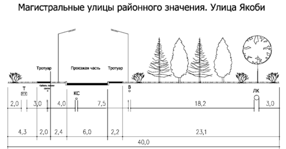
1.4. Поперечные профили улиц и магистралей
