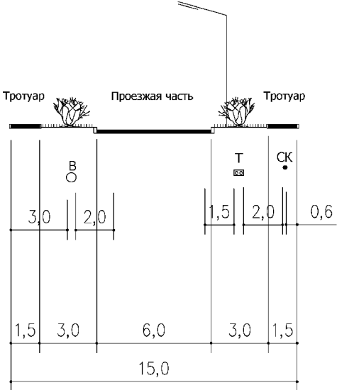
Улица местного значения. ул. Одесская (сечение разреза 6-6)
