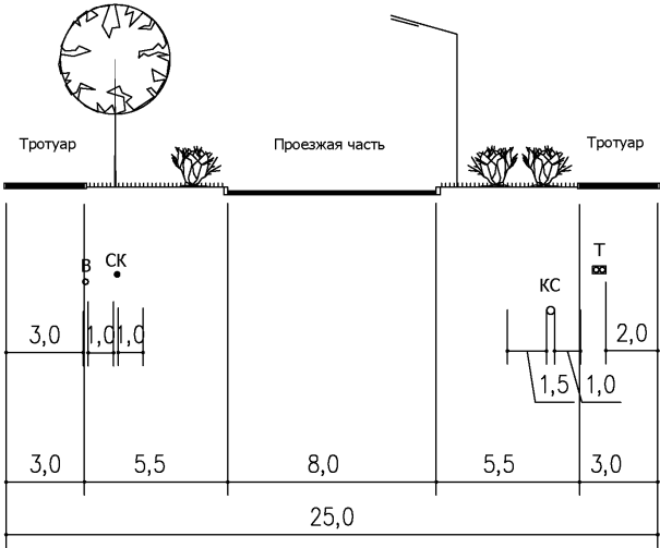
Улица местного значения. ул. Одесская (сечение разреза 6-6)
