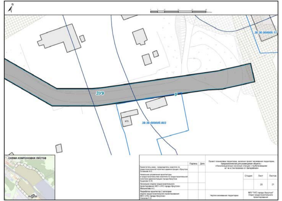
ПРОЕКТ ПЛАНИРОВКИ ТЕРРИТОРИИ, ВКЛЮЧАЯ ПРОЕКТ МЕЖЕВАНИЯ ТЕРРИТОРИИ, ПРЕДНАЗНАЧЕННОЙ ДЛЯ РАЗМЕЩЕНИЯ ЛИНЕЙНОГО ОБЪЕКТА — «КАНАЛИЗАЦИОННЫЕ НАСОСНЫЕ СТАНЦИИ С ТРУБОПРОВОДАМИ В 1-М И 2-М ПОСЕЛКАХ СТ. БАТАРЕЙНАЯ»
