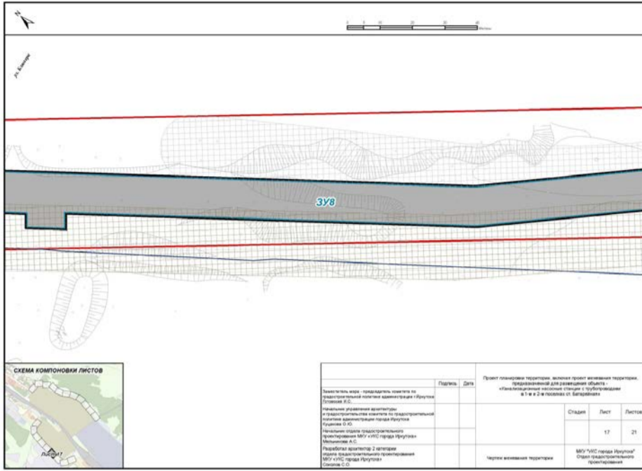
ПРОЕКТ ПЛАНИРОВКИ ТЕРРИТОРИИ, ВКЛЮЧАЯ ПРОЕКТ МЕЖЕВАНИЯ ТЕРРИТОРИИ, ПРЕДНАЗНАЧЕННОЙ ДЛЯ РАЗМЕЩЕНИЯ ЛИНЕЙНОГО ОБЪЕКТА — «КАНАЛИЗАЦИОННЫЕ НАСОСНЫЕ СТАНЦИИ С ТРУБОПРОВОДАМИ В 1-М И 2-М ПОСЕЛКАХ СТ. БАТАРЕЙНАЯ»
