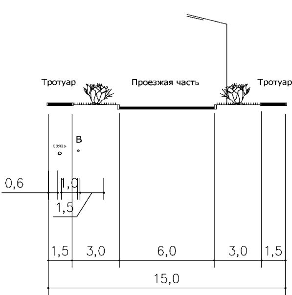
УЛИЦА МЕСТНОГО ЗНАЧЕНИЯ (СЕЧЕНИЕ РАЗРЕЗА 7-7)
