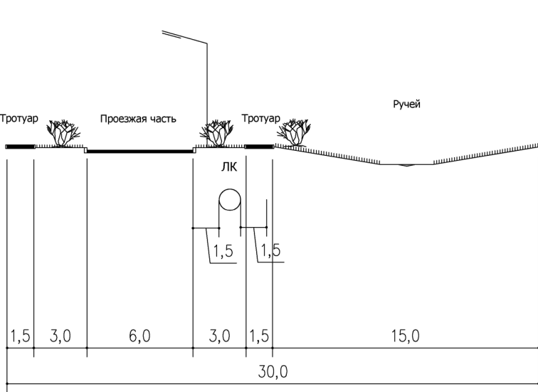
УЛИЦА МЕСТНОГО ЗНАЧЕНИЯ (СЕЧЕНИЕ РАЗРЕЗА 8-8)
