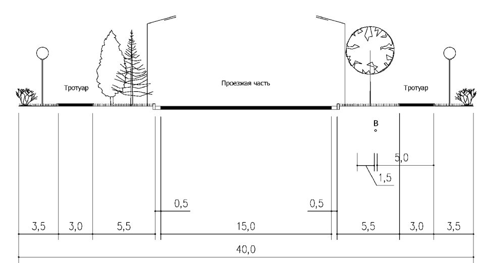
МАГИСТРАЛЬНАЯ УЛИЦА ОБЩЕГОРОДСКОГО ЗНАЧЕНИЯ РЕГУЛИРУЕМОГО ДВИЖЕНИЯ УЛ. ФРУНЗЕ (СЕЧЕНИЕ РАЗРЕЗА 3-3)
