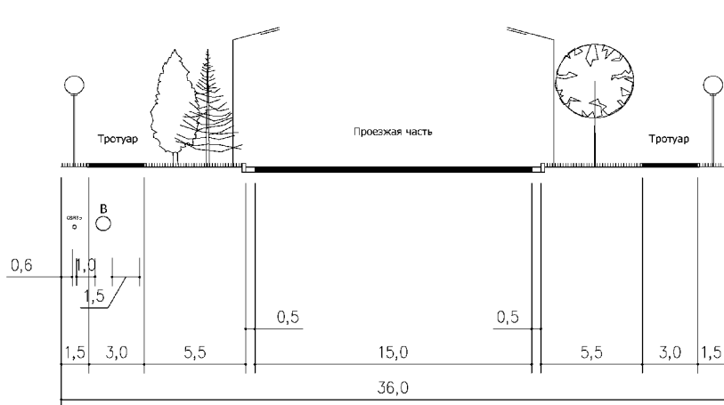
МАГИСТРАЛЬНАЯ УЛИЦА РАЙОННОГО ЗНАЧЕНИЯ (СЕЧЕНИЕ РАЗРЕЗА 6-6)
