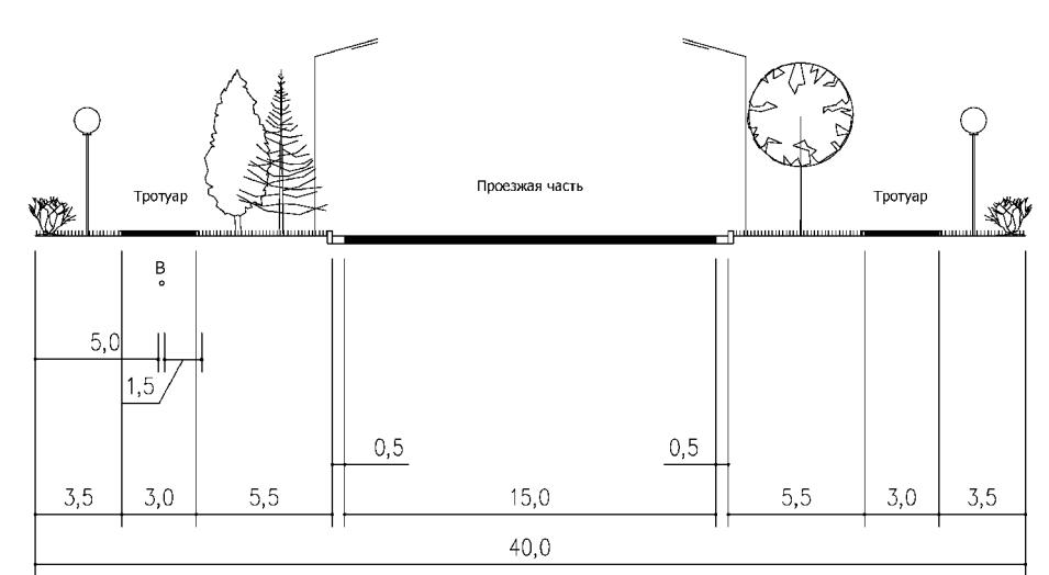
МАГИСТРАЛЬНАЯ УЛИЦА РАЙОННОГО ЗНАЧЕНИЯ. УЛИЦА ПЕРВОМАЙСКАЯ (СЕЧЕНИЕ РАЗРЕЗА 2-2)
