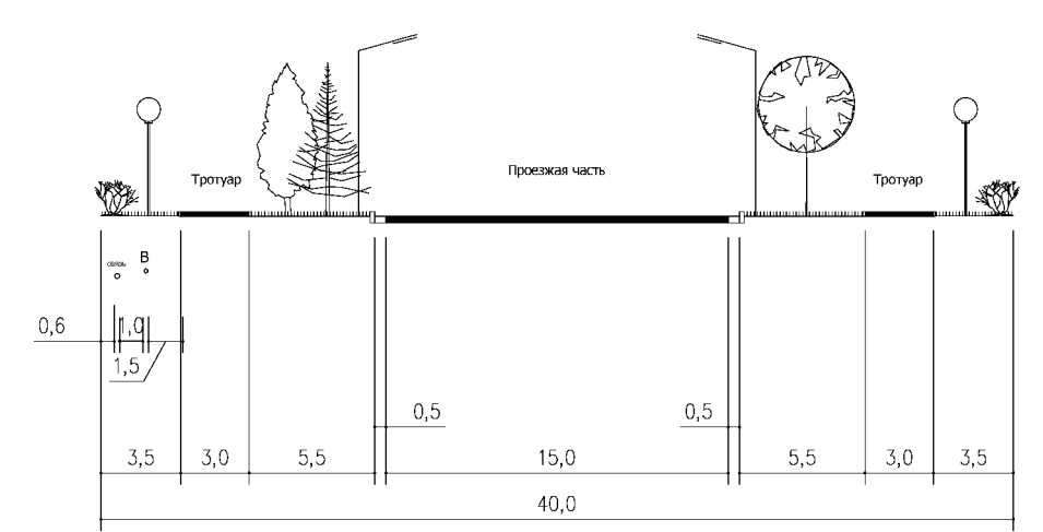
1.3. ПОПЕРЕЧНЫЕ ПРОФИЛИ УЛИЦ И ДОРОГ В КРАСНЫХ ЛИНИЯХ МАГИСТРАЛЬНАЯ УЛИЦА РАЙОННОГО ЗНАЧЕНИЯ. УЛИЦА ПЕРВОМАЙСКАЯ (СЕЧЕНИЕ РАЗРЕЗА 1-1)
