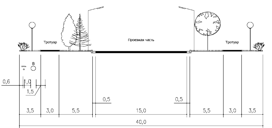
МАГИСТРАЛЬНАЯ УЛИЦА ОБЩЕГОРОДСКОГО ЗНАЧЕНИЯ РЕГУЛИРУЕМОГО ДВИЖЕНИЯ УЛ. СЕВЕРНАЯ (СЕЧЕНИЕ РАЗРЕЗА 5-5)
