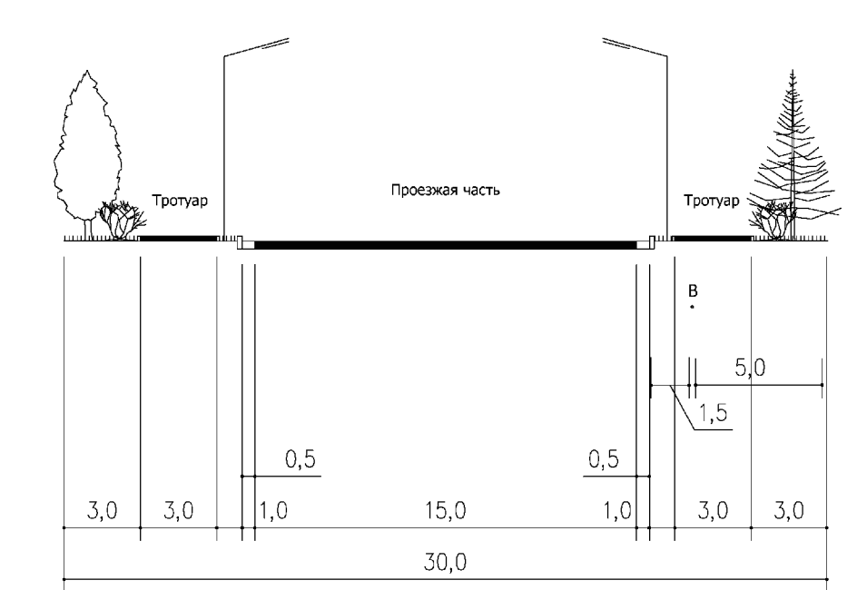
МАГИСТРАЛЬНАЯ УЛИЦА ОБЩЕГОРОДСКОГО ЗНАЧЕНИЯ РЕГУЛИРУЕМОГО ДВИЖЕНИЯ УЛ. МЕЛЬНИЧНАЯ (СЕЧЕНИЕ РАЗРЕЗА 4-4)
