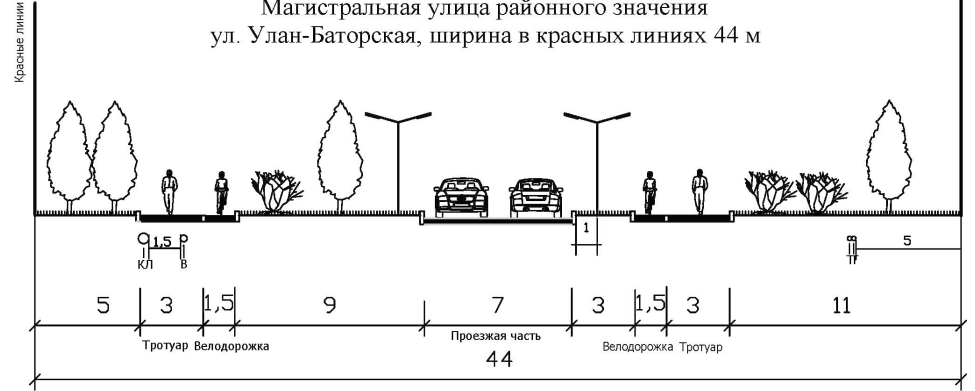
РАЗРЕЗ 2-2
