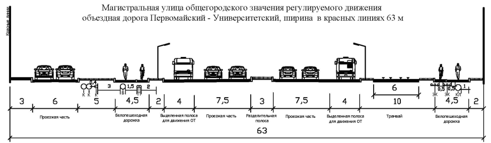
РАЗРЕЗ 1-1
