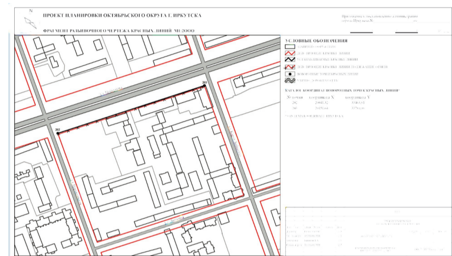
Проект планировки Октябрьского округа г. Иркутска Фрагмент разбивочного чертежа красных линий М 1:2000
