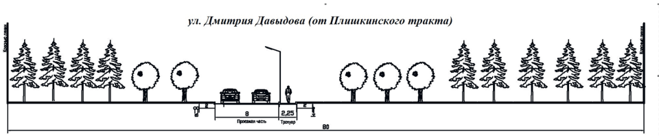
ПОПЕРЕЧНЫЕ ПРОФИЛИ УЛИЦ И ДОРОГ В КРАСНЫХ ЛИНИЯХ РАЗРЕЗ 1-1
