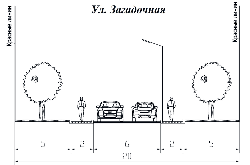
РАЗРЕЗ 4-4
