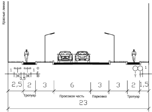
Улица местного значения ул. Коммунистическая, ширина в красных линиях 23 м
