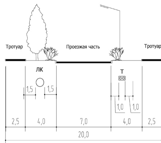
МАГИСТРАЛЬНАЯ УЛИЦА РАЙОННОГО ЗНАЧЕНИЯ. УЛИЦА КАШТАКОВСКАЯ (СЕЧЕНИЕ РАЗРЕЗА 7-7)
