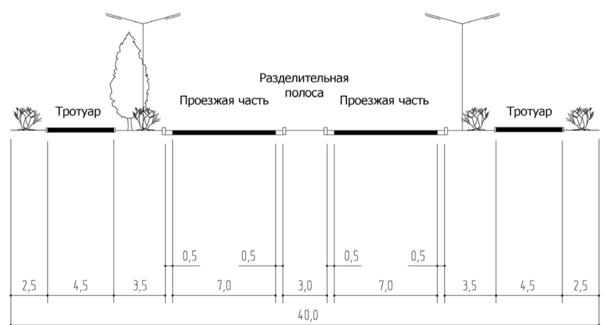
МАГИСТРАЛЬНАЯ УЛИЦА РАЙОННОГО ЗНАЧЕНИЯ. УЛИЦА ФУЧИКА (СЕЧЕНИЕ РАЗРЕЗА 8-8)
