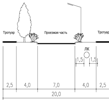
Магистральная улица районного значения. Ул. Напольная 2-2
