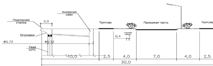
Улицы местного значения. 3-3
