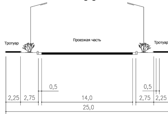
Магистральные улицы районного значения. Улица Напольная 5-5
