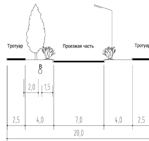
МАГИСТРАЛЬНАЯ УЛИЦА РАЙОННОГО ЗНАЧЕНИЯ. УЛИЦА ФУЧИКА (СЕЧЕНИЕ РАЗРЕЗА 8-8)
