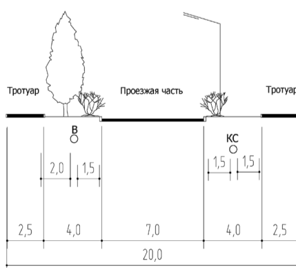
МАГИСТРАЛЬНАЯ УЛИЦА РАЙОННОГО ЗНАЧЕНИЯ. УЛИЦА НАПОЛЬНАЯ (СЕЧЕНИЕ РАЗРЕЗА 5-5)
