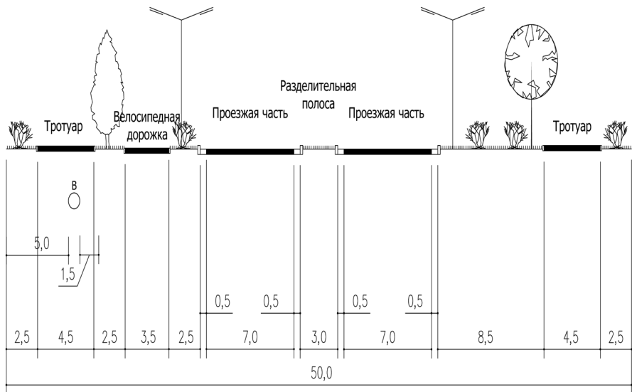
РЕКОНСТРУКЦИЯ МАГИСТРАЛЬНОЙ УЛИЦЫ ОБЩЕГОРОДСКОГО ЗНАЧЕНИЯ РЕГУЛИРУЕМОГО ДВИЖЕНИЯ УЛ. СТАРОКУЗЬМИХИНСКАЯ ШИРИНА В КРАСНЫХ ЛИНИЯХ — 50 М. (СЕЧЕНИЕ РАЗРЕЗА 11-11)
