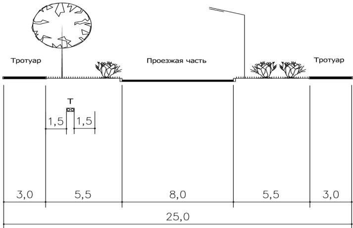
УЛИЦА МЕСТНОГО ЗНАЧЕНИЯ ПРОБИВКА ОТ УЛ. ЛЕРМОНТОВА ДО УЛ. МАЙСКАЯ ШИРИНА В КРАСНЫХ ЛИНИЯХ — 15-25 М. (СЕЧЕНИЕ РАЗРЕЗА 9-9)
