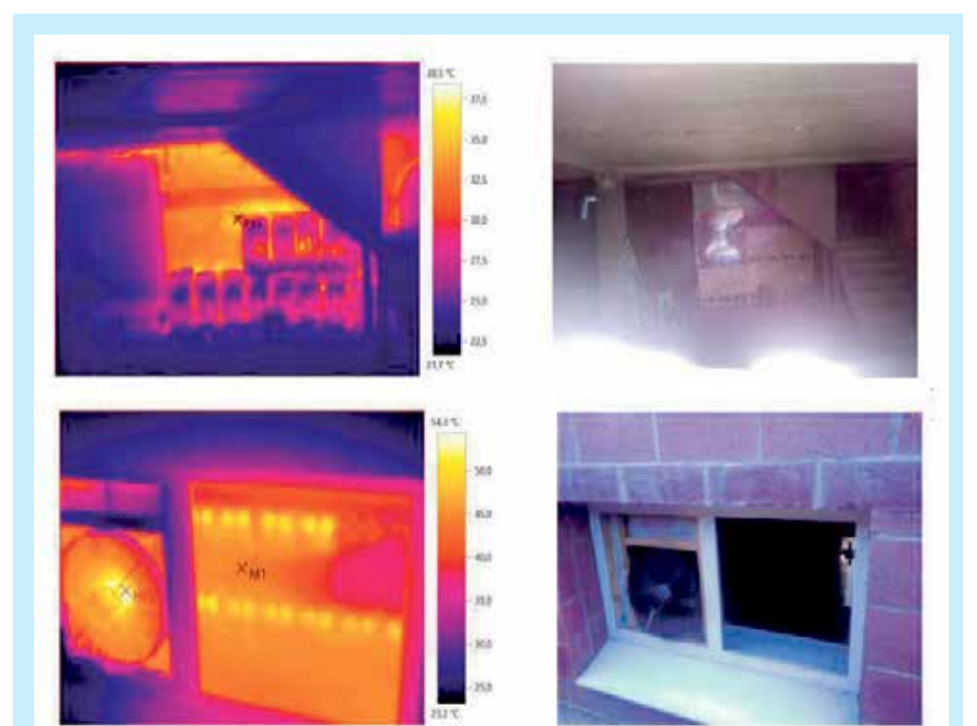
Вот так на тепловизоре выглядит помещение, где работают машинки для добычи криптовалюты. Температура воздуха вокруг асиков* достигает 37–45 градусов по Цельсию
